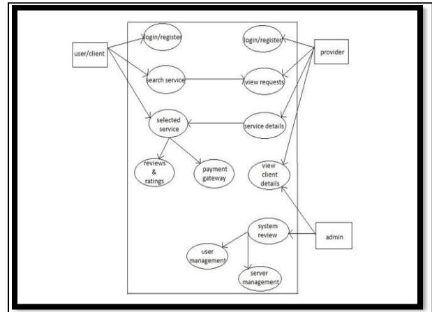
Figure 2 ER Diagram
