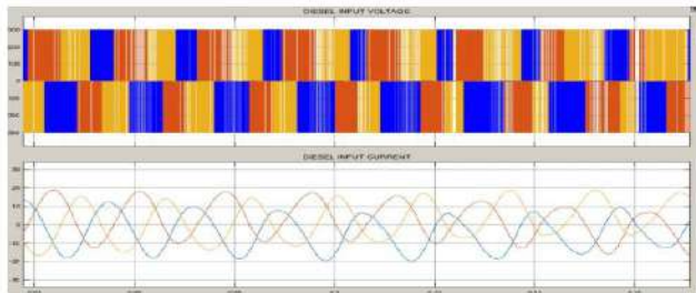
Fig.21. Diesel Input.
