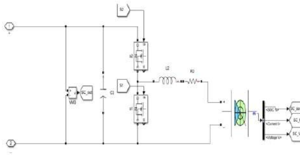
Fig.6. Super Capacitor.
