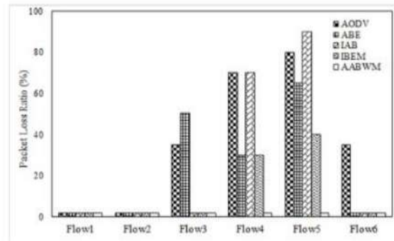
Fig. 4.11. Packet loss ratio.
